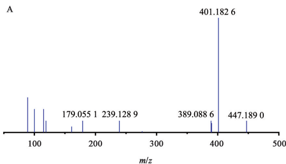
注:A.质谱图;B.裂解规律图(图2-图6同)
